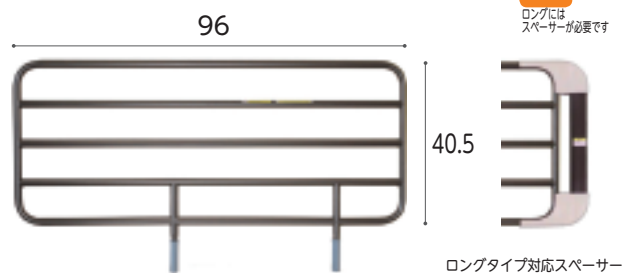
ロングタイプ対応スペーサー (取付時サイズ幅 103×高さ 40.5)
